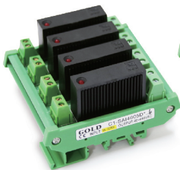
4路(5A) 卡座式安装
